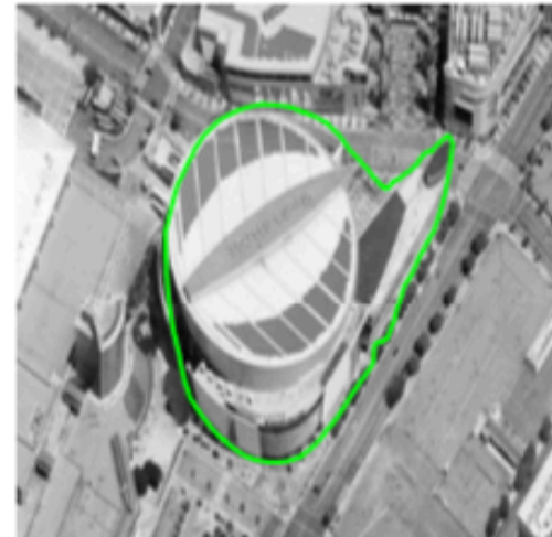
(d) Result
